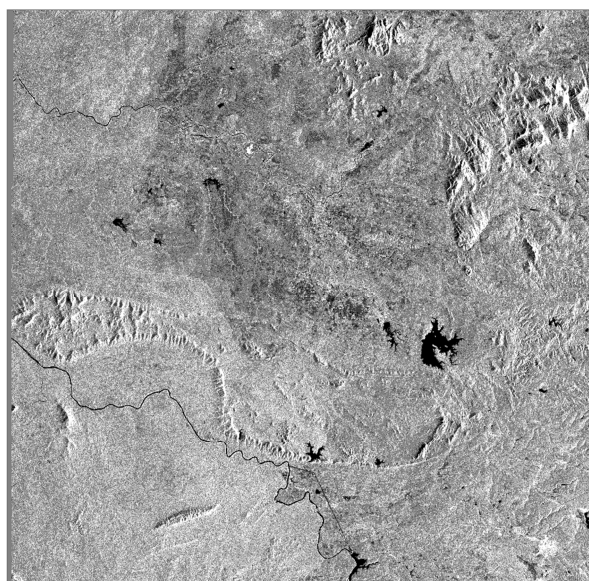
NDVI VV
