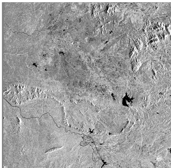
NDVI VV+VH
